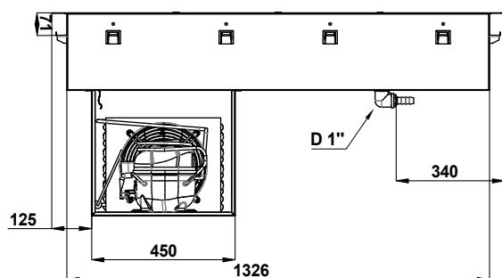
Zij aanzicht
